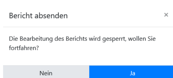
Abbildung 65: Bericht absenden
