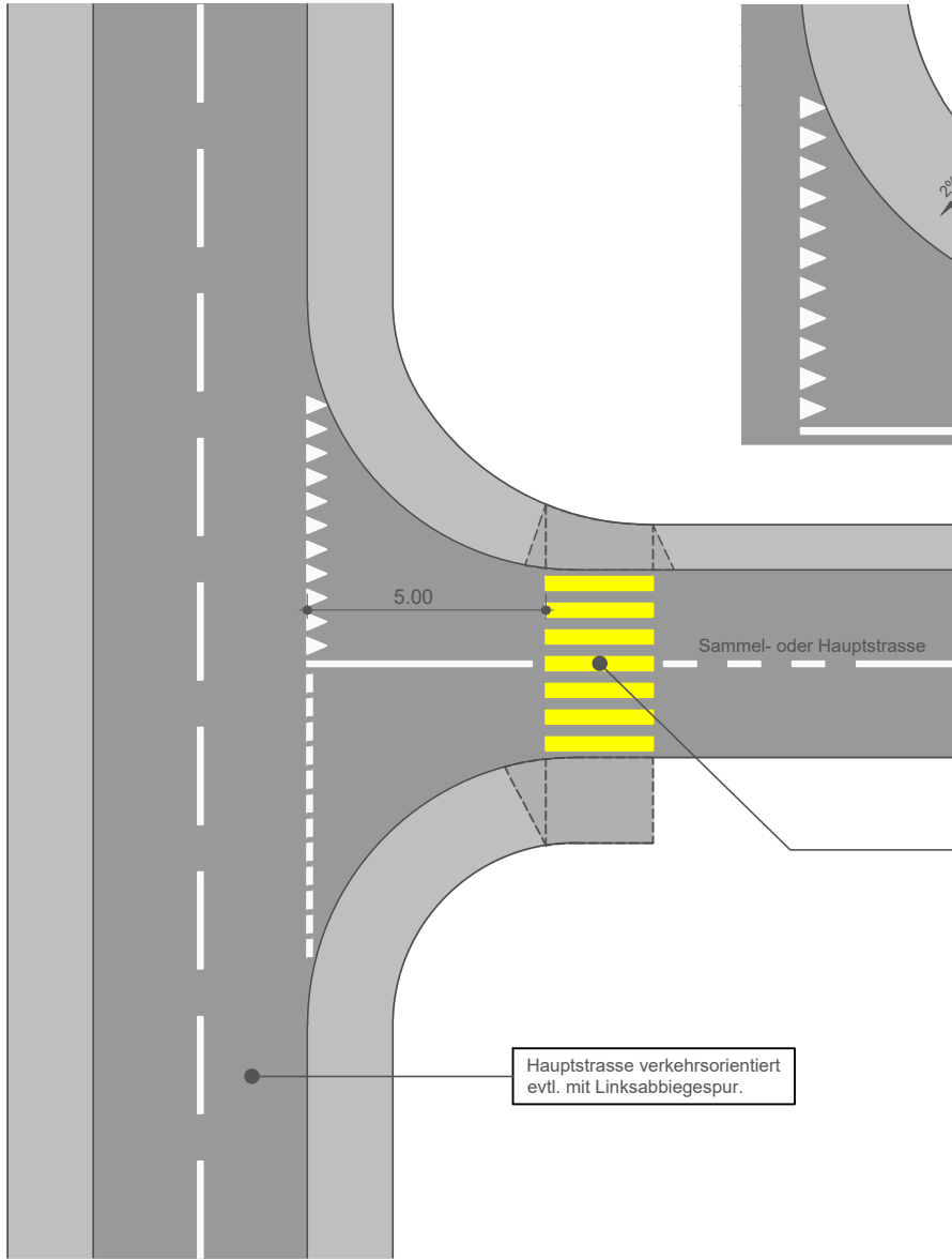
Detail Trottoirabsenkung
