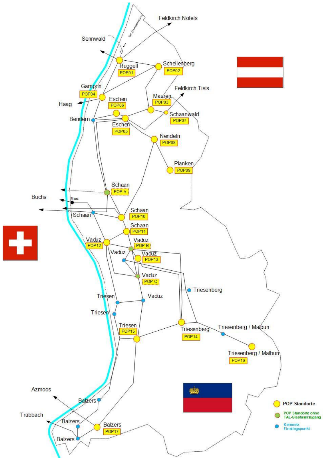
Abbildung 2 Anschlusszentralen LKW
