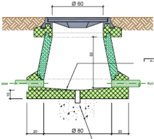
Abbildung 10 Kabelkanalisation: Kontrollschacht
