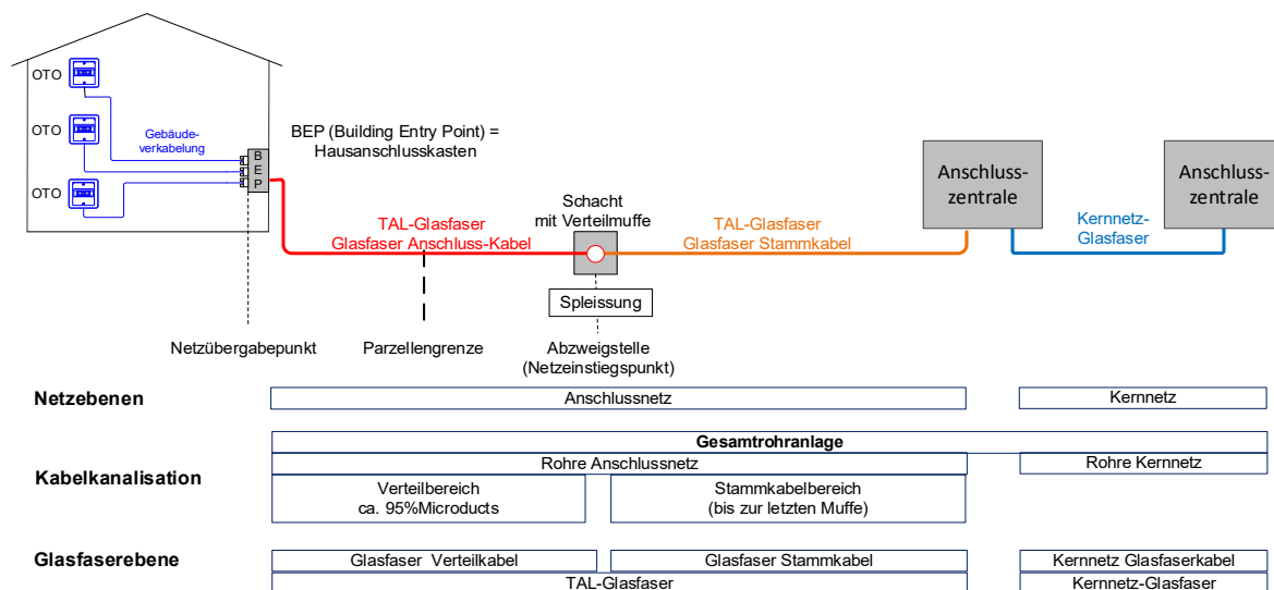
Abbildung 3 Kabelkanalisation: Netzschema
