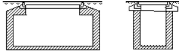
Abbildung 7 Kabelkanalisation: Kleineinstiegschacht
