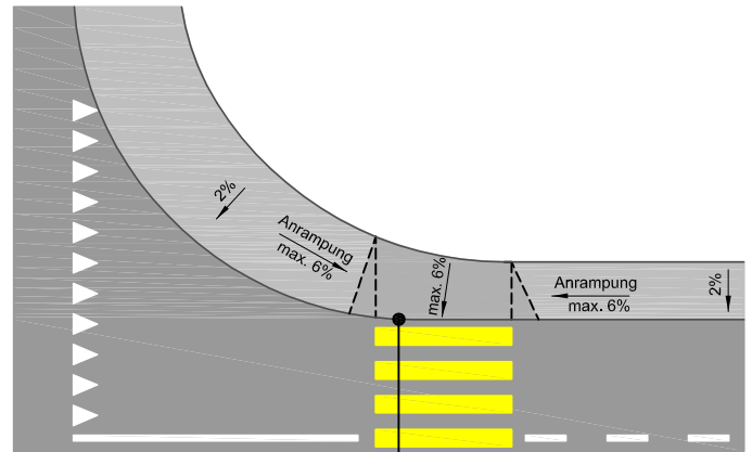
Detail Trottoirabsenkung
